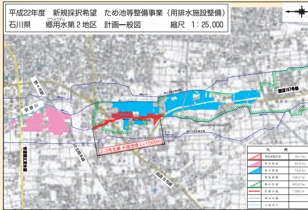
計画位置図
