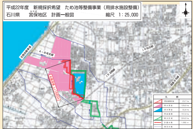
計画位置図
